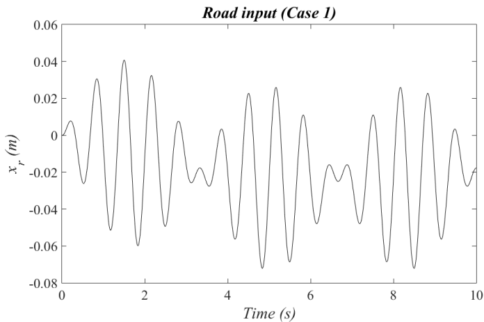
Fig3.Road input case 1 [12].
