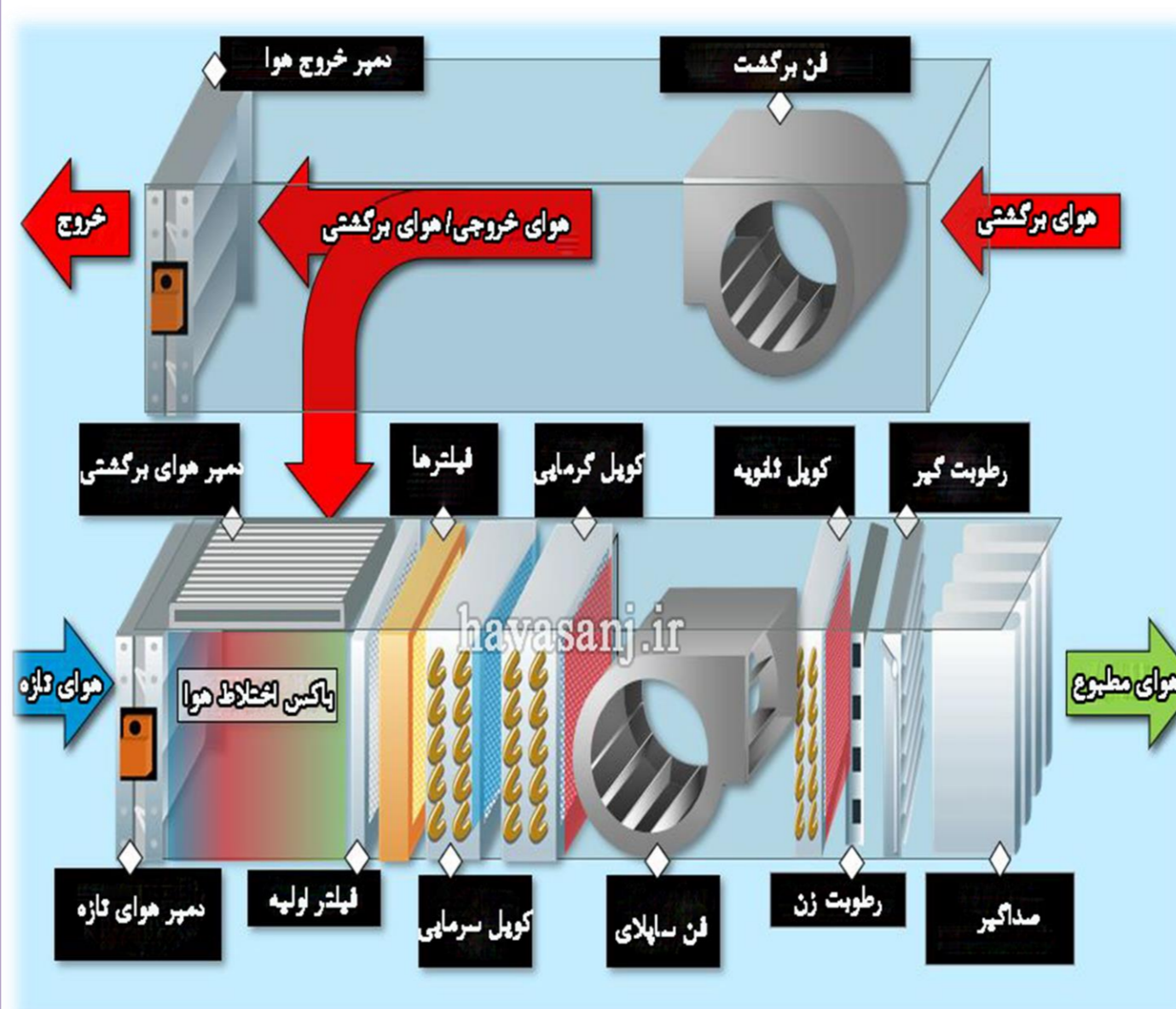
شکل ۱ اجزای مختلف دستگاه هواساز
